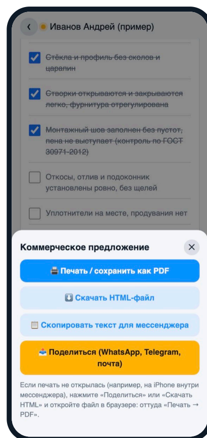
Окно выгрузки.
