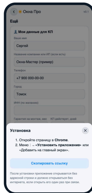
Окно «Установка».
