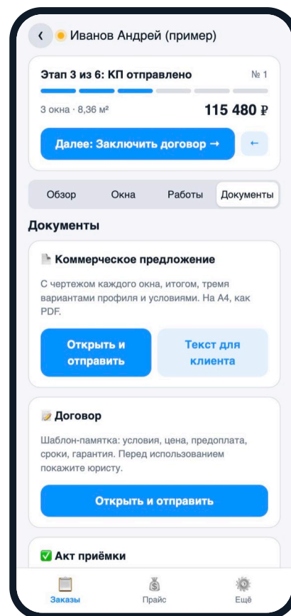
Карточки документов.
